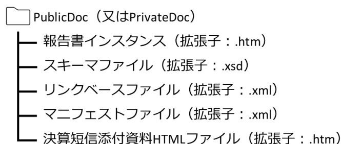
図 3-1 決算短信財務諸表 XBRL ファイルのフォルダ構成
